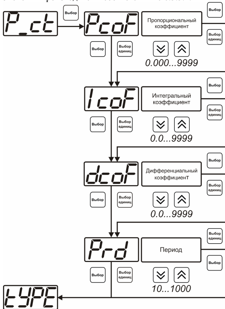
Рисунок 6.22 Настройка коэффициентов ПИД-регулятора (реле)
