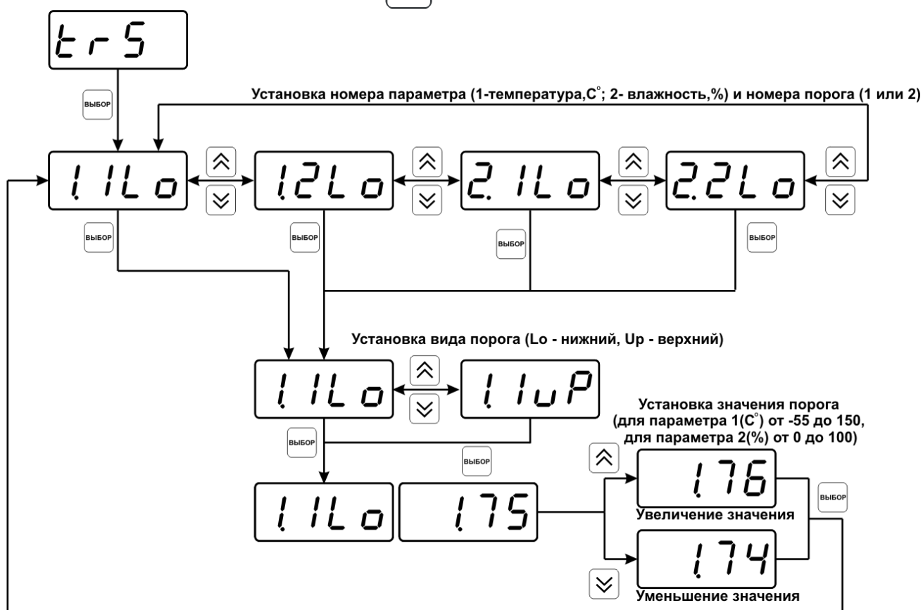
Рисунок 6.11 Задание порогов по влажности и температуре
