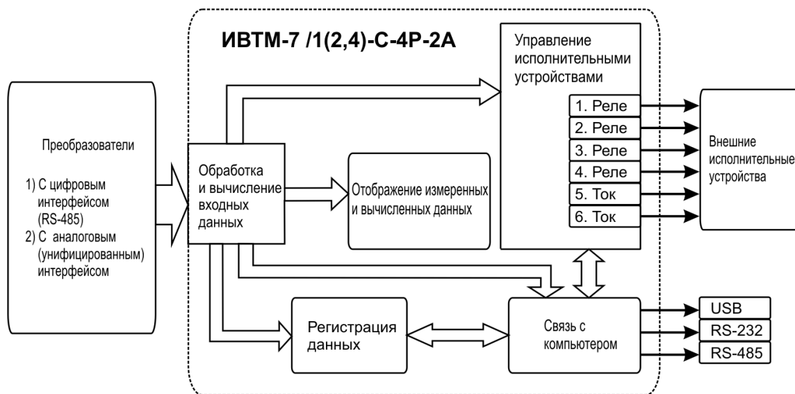
Рисунок 3.9 Структурная схема работы прибора
