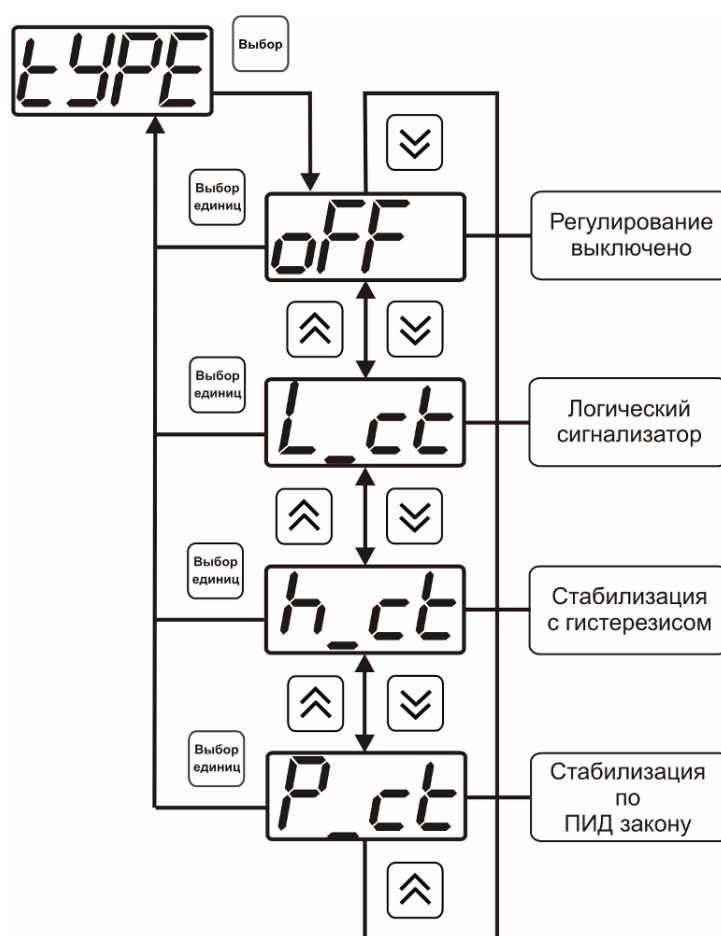
Рисунок 6.17 Выбор логики работы канала управления (реле)
